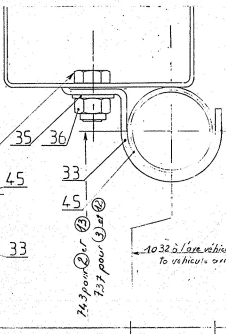
COUPE K K SECTION
