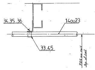
COUPE RR SECTION
