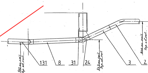
COUPE X X SECTION
