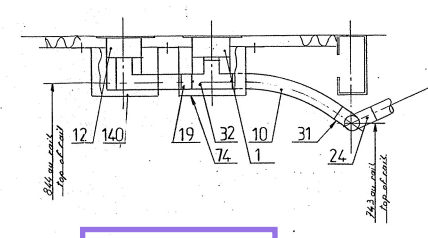
COUPE YY SECTION
