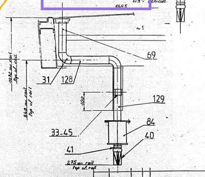
COUPE GG SECTION
